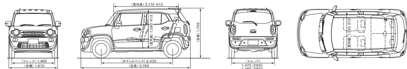
寸法図(HYBRID MZ)単位:mm
