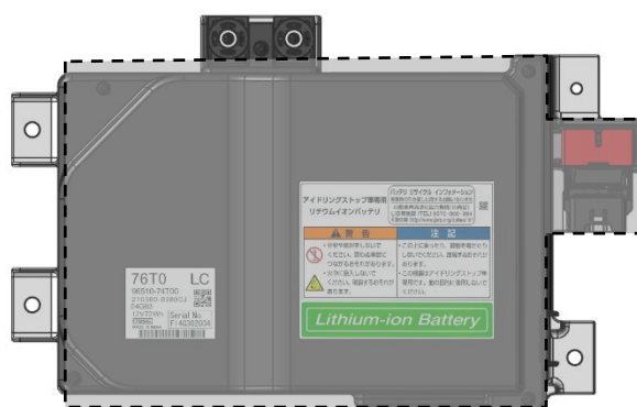
C. マイルドハイブリッド用 72Wh LiB パック
