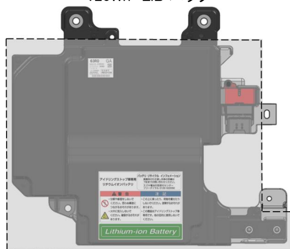
D. マイルドハイブリッド用 120Wh LiB パック
