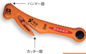
万が一の事故の際や水没時など、車内に閉じ込められてしまった際に、 シートベルトを切断し、サイドウィンドウを破砕して車外へ 脱出するための緊急脱出用ハンマーです。
