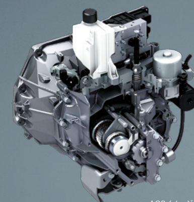
AGSイメージ図
