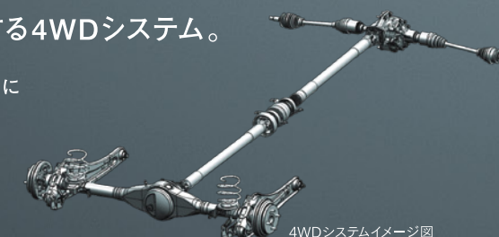
4WDシステムイメージ図
