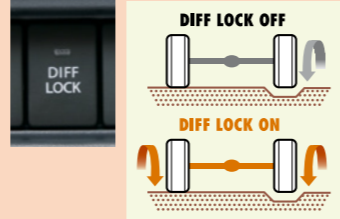
ぬかるみなどで後輪の片方が空回りした場合に、スイッチをONにするだけで、もう一方のタイヤに駆動力を伝達。ぬかるみなどからの脱出時に威力を発揮します。 *デフロック機構は、安全のため30km/hを超えた場合は自動的に解除されます。
