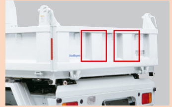
負荷のかかりやすい部分を強化するために、サイドゲート、リヤゲートに補強柱を装着。
