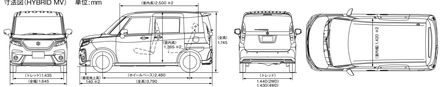
寸法図(HYBRID MV) 単位:mm
