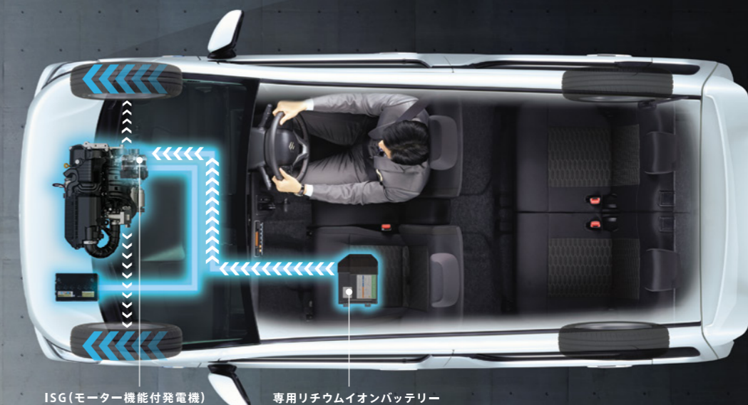
ISG (モーター機能付発電機) 専用リチウムイオンバッテリー
