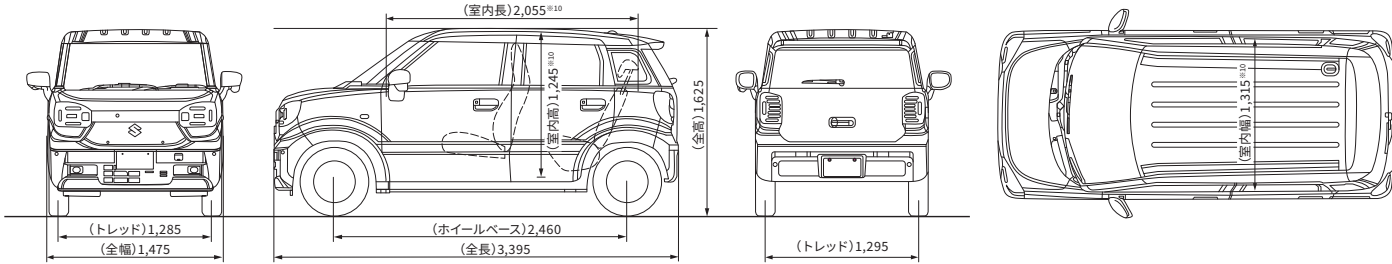
寸法図 (X) 単位:mm
