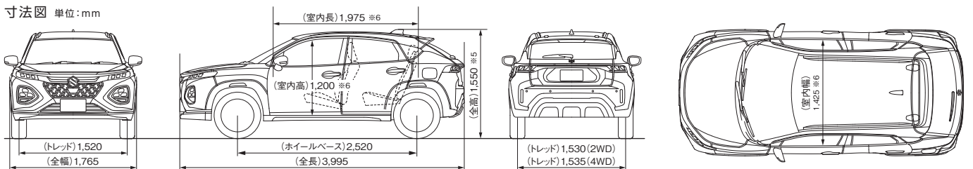
寸法図 単位:mm
