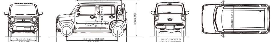
寸法図 (HYBRID X) 単位:mm
