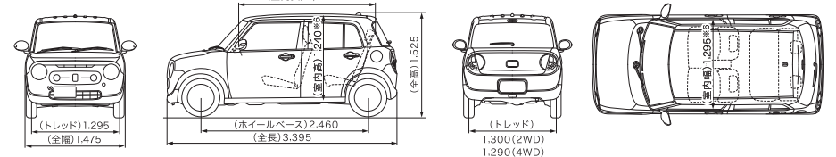
寸法図 (X) 単位: mm
