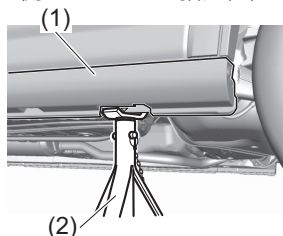
リヤ側リジッドラック指定位置
