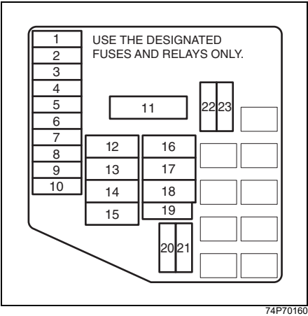
リレーボックス No.1
