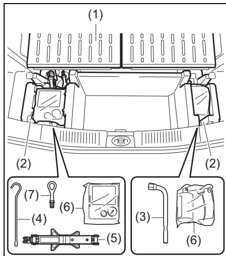
2WD車
