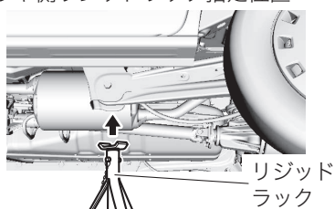
リア側リジッドラック指定位置
