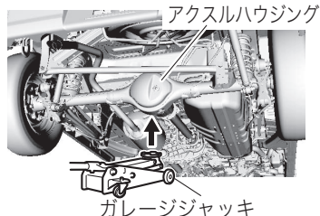
リア側ガレージジャッキ指定位置
