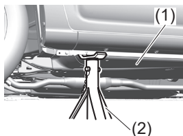
フロント側リジッドラック指定位置
