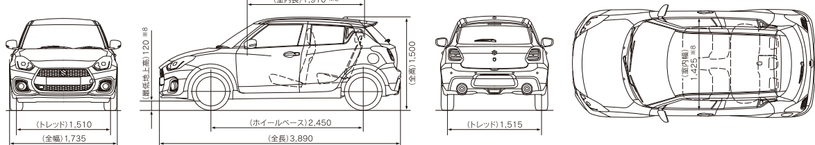
寸法図 単位:mm
