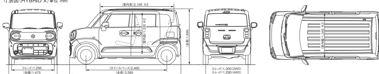
寸法図(HYBRID X)単位:mm
