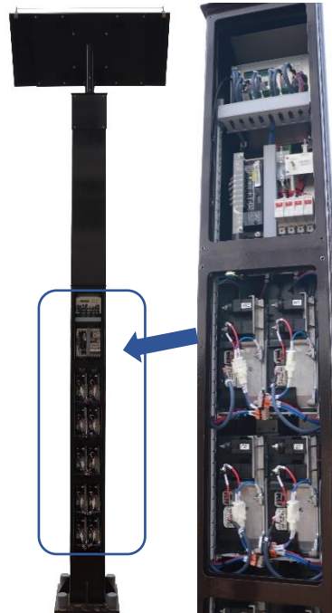
リチウムイオン電池を内蔵した 街灯の内部
